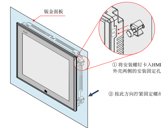
图3 安装示意图
